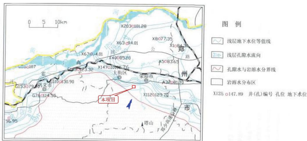
图 4.2-2 荥阳市地下水水位等值线图
