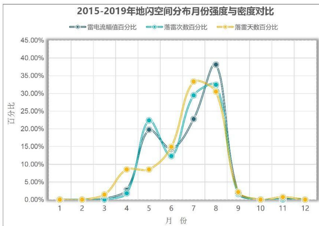
图 4.2-7 项目所在地 2015 年至 2019 年地闪空间分布月份对比图
