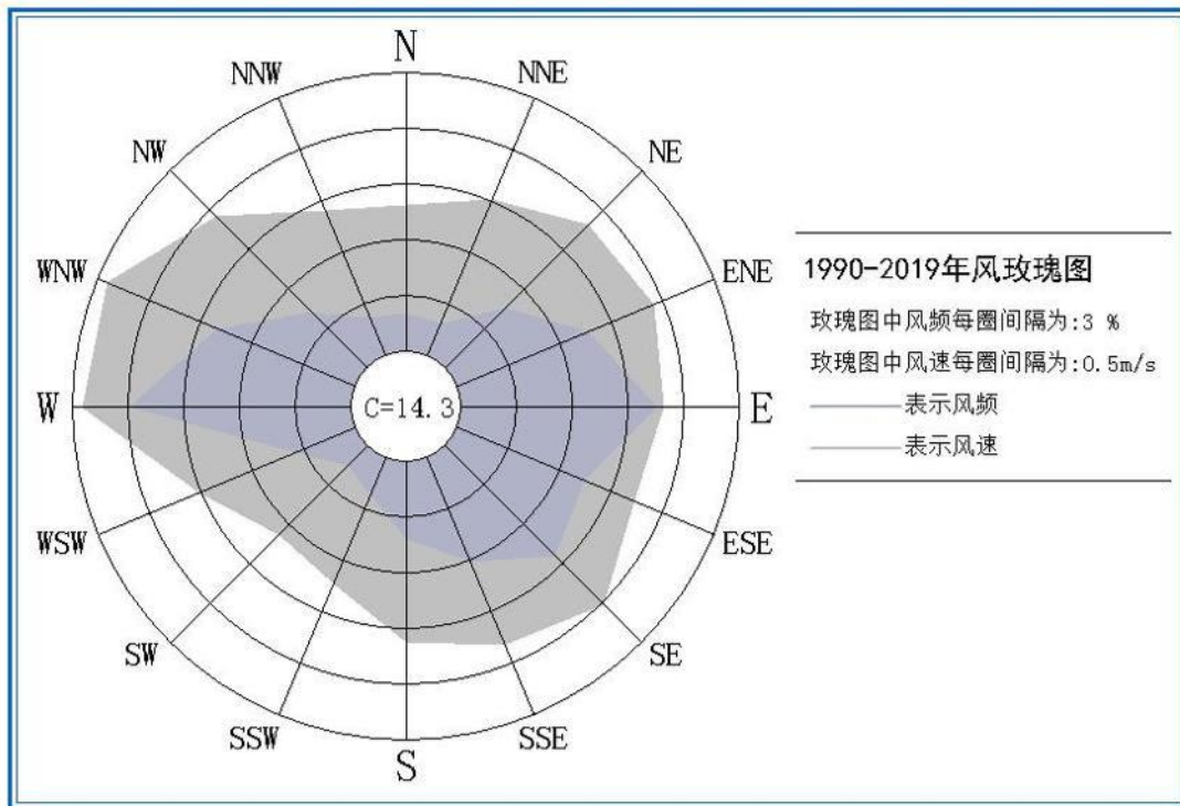
图 3.7-3 1990-2019 年荃阳站风向风速玫瑰图
