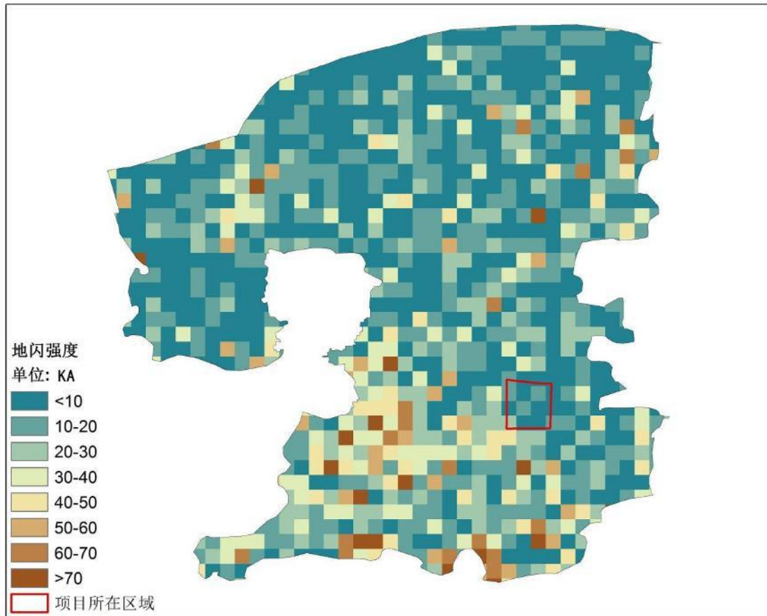
图 4.4-5 郑东新区核心板块地闪强度图
