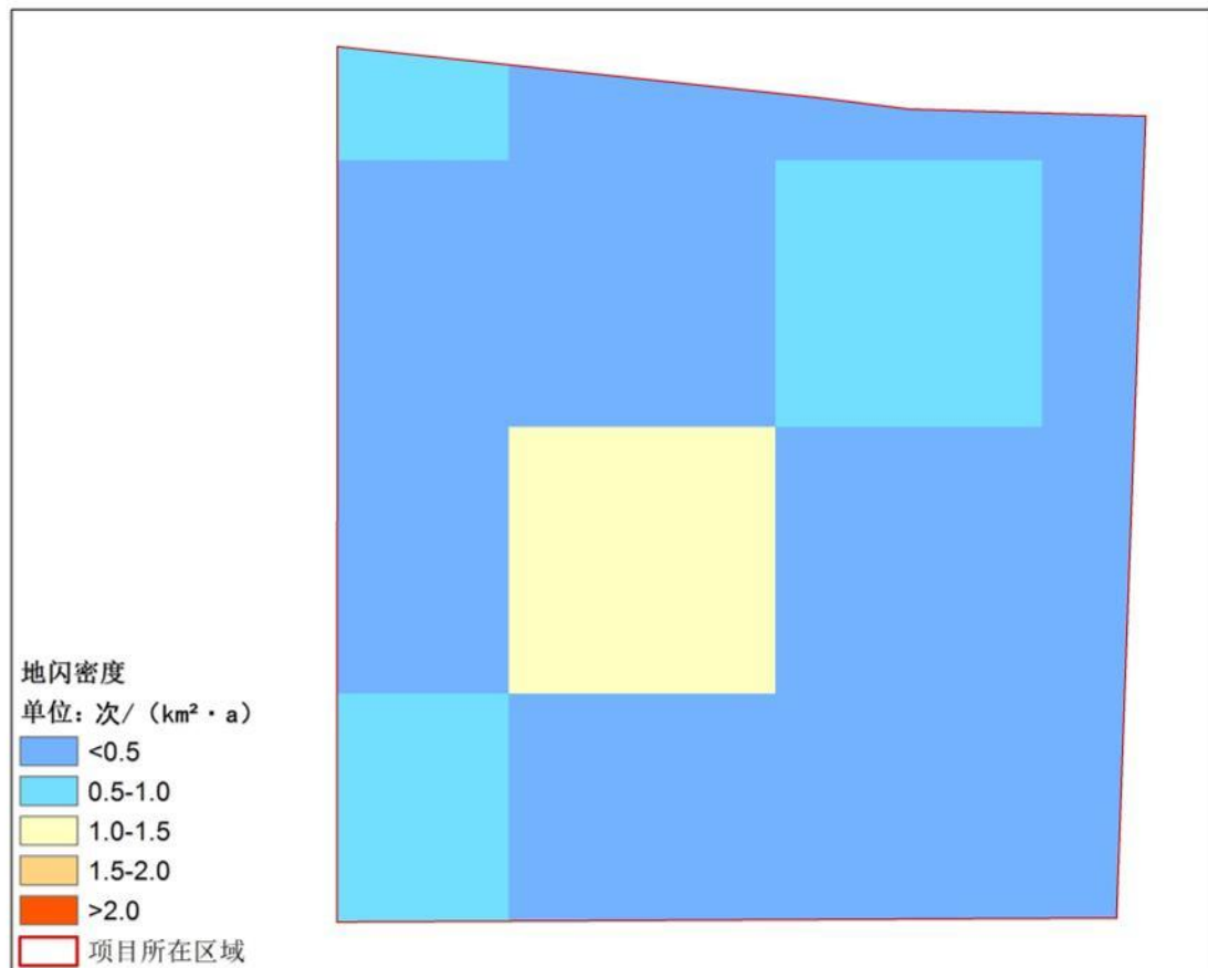
图 4.4-3 荥阳市宜居健康示范区域地闪密度分布图 (格点 1km×1km)
