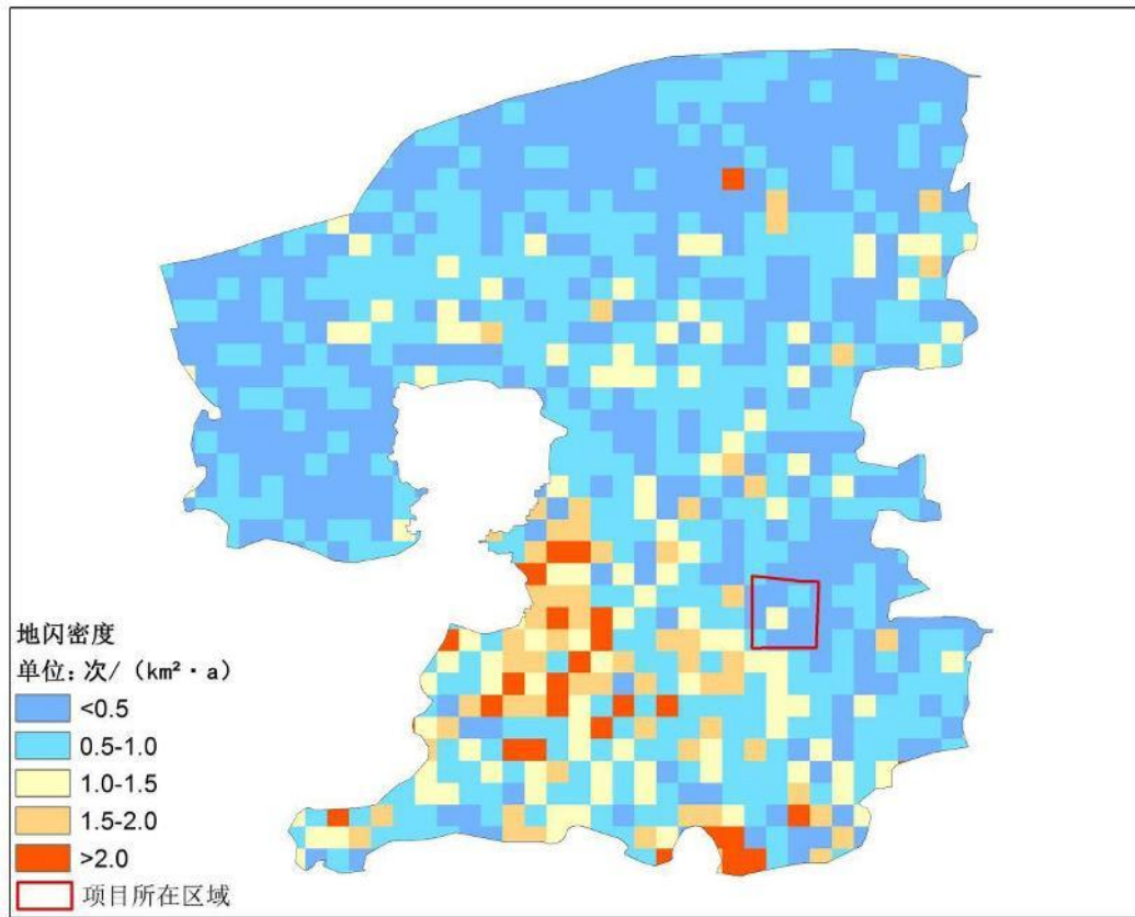
图 4.4-2 荥阳市宜居健康示范区地闪密度图
