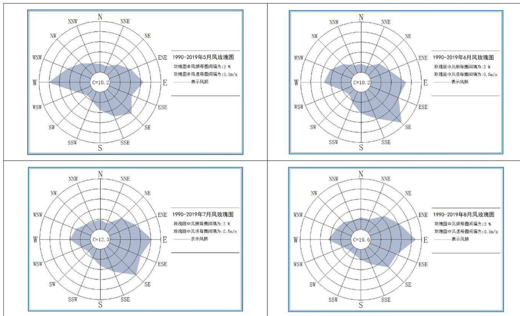
图 3.7-6 1990-2019 年荃阳站 5-8 月份平均风向频率玫瑰图
