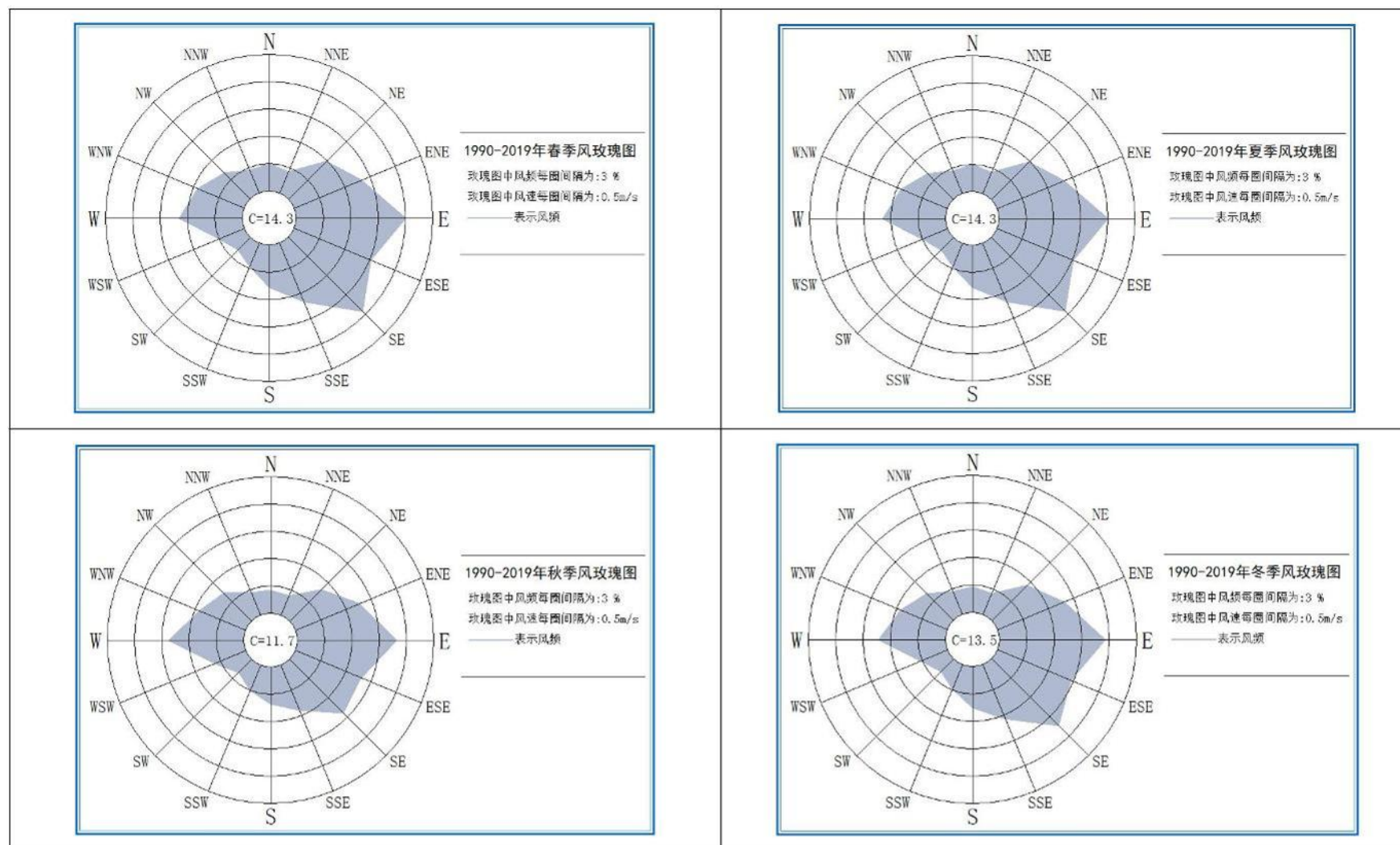
图 3.7-4 1990—2019 年荥阳各季节平均风向频率玫瑰图
